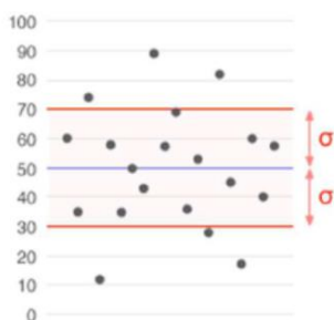
Una serie di dati con una media di 50 (in blu) ed una deviazione standard ( \sigma ) di 20.
